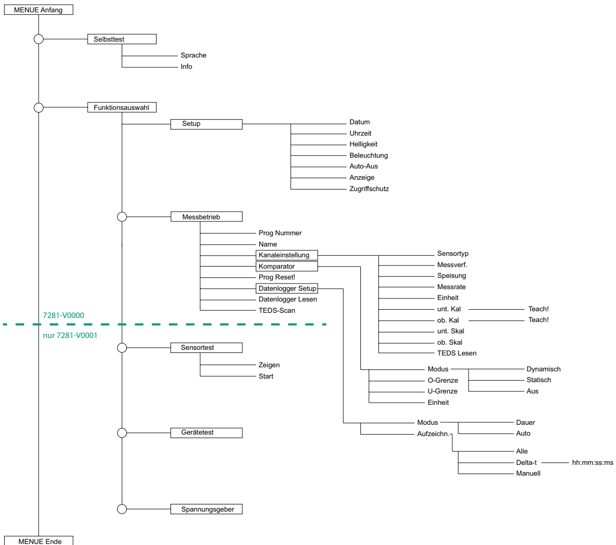
Abbildung 5: Menüstruktur TRANS CAL Typ 7281-V0001
