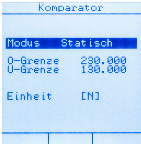
Abbildung 13: Komparatoreinstellung
