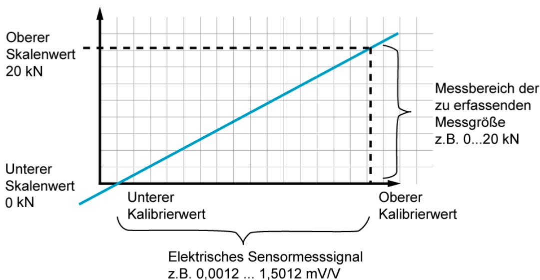
Abbildung 11: Skalierung und Kalibrierwert
