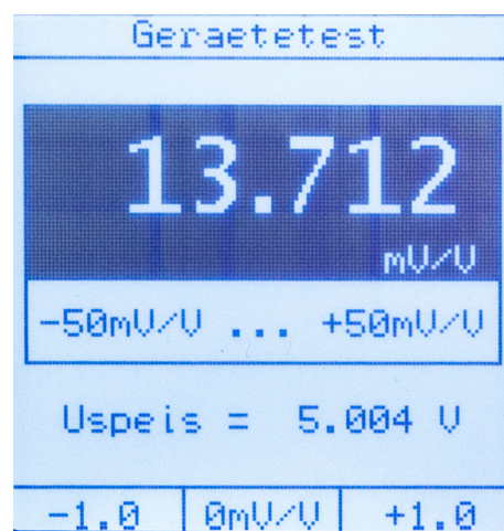
Abbildung 22: Funktion „Gerätetest“, Bereich \pm 50 mV/V
